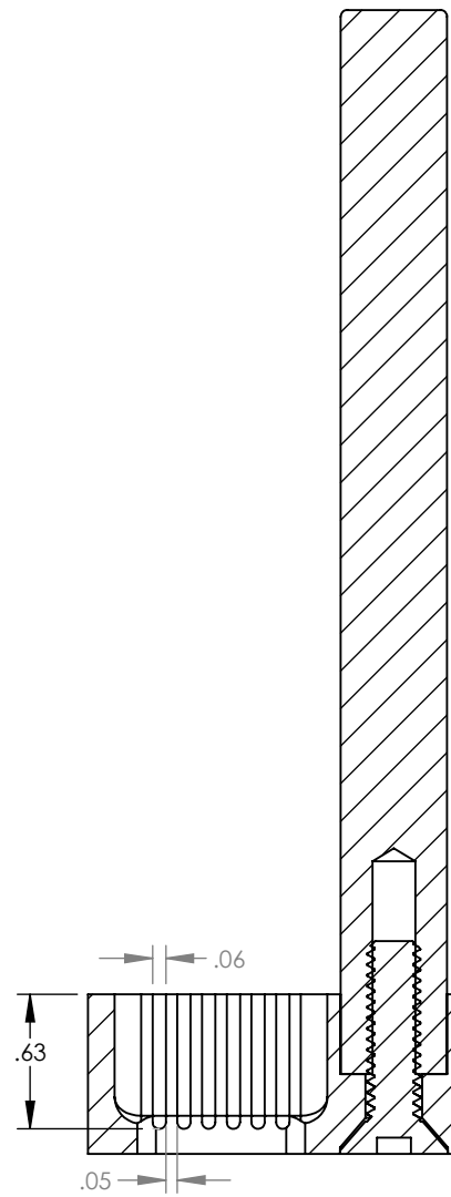
SECTION A-A SCALE 1 : 1
